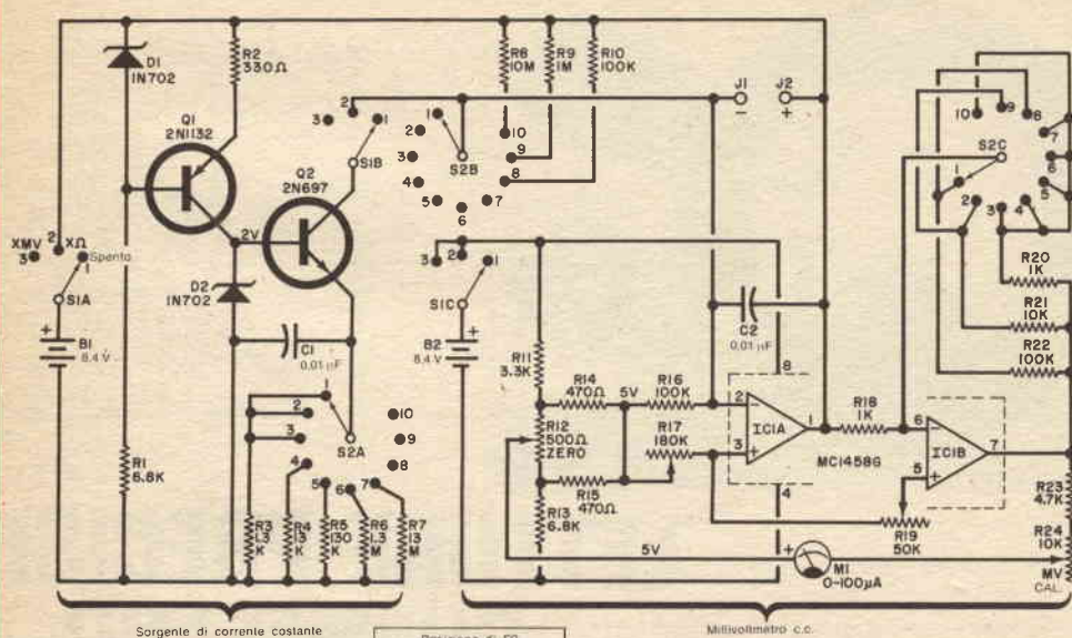
Sorgente di corrente costante
